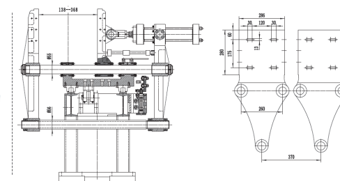
HTS II-2L (挤出中空吹塑设备)
